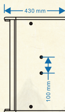
侧视图
