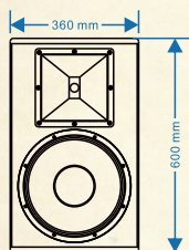
主视图
